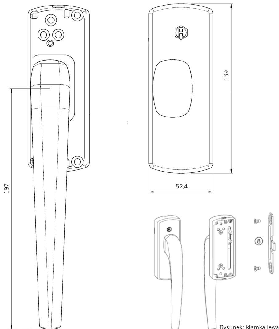
Rysunek: klamka lewa
